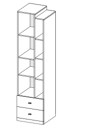
пенал П-1 450x2220x420
