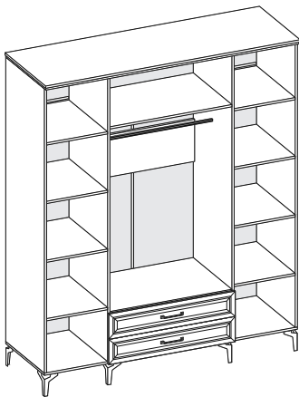
шкаф ШК-4 1810x2220x580
