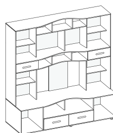
центральная секция 2150x2094x520
