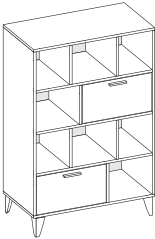
комод К-1 800x1196/1241x408
