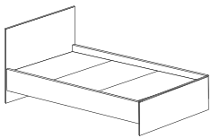
кровать арт. 032 0,9 с низким щитком 950x800x2032
