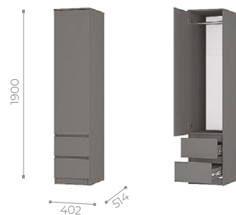
Пенал «Симпл» (ПН-17) (можно доукомплектовать полками ПЛ-05)
