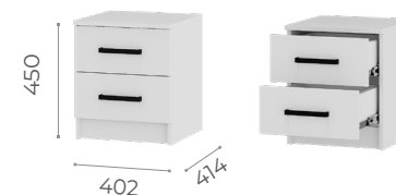
ТУМБА ПРИКРОВАТНАЯ (ТБ-12) (шариковые направляющие)
