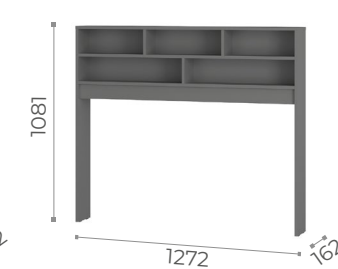
Стеллаж-полка «Симпл» (СП-03) (можно использовать как надстройку к кровати КР-07)
