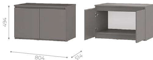
Тумба «Симпл» (ТБ-06) (можно использовать как антресоль к ШК-03)
