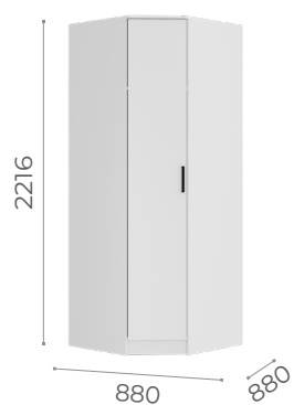
ШКАФ УГЛОВОЙ (ШКУ-04) (универсальная сборка)
