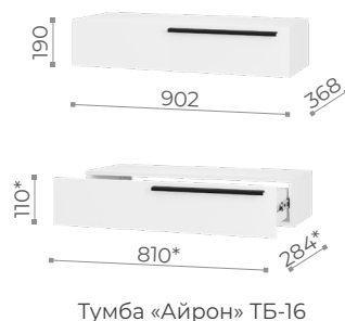
Тумба «Айрон» ТБ-16
