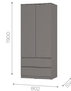
Шкаф 2-х створчатый «Симпл» (ШК-03) (универсальная сборка)
