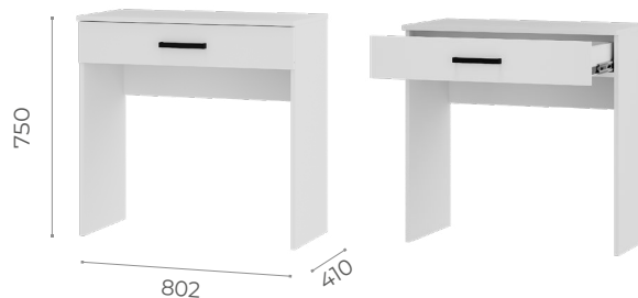
СТОЛ ТУАЛЕТНЫЙ (СТ-02) (шариковые направляющие)
