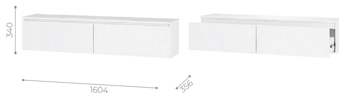
Шкаф навесной «Симпл» (ШКН-07)
